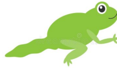
froglet
